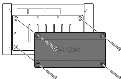
図 1 バッテリーケースの取り付け方
