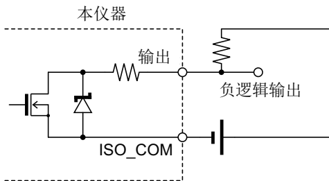
负逻辑输出
