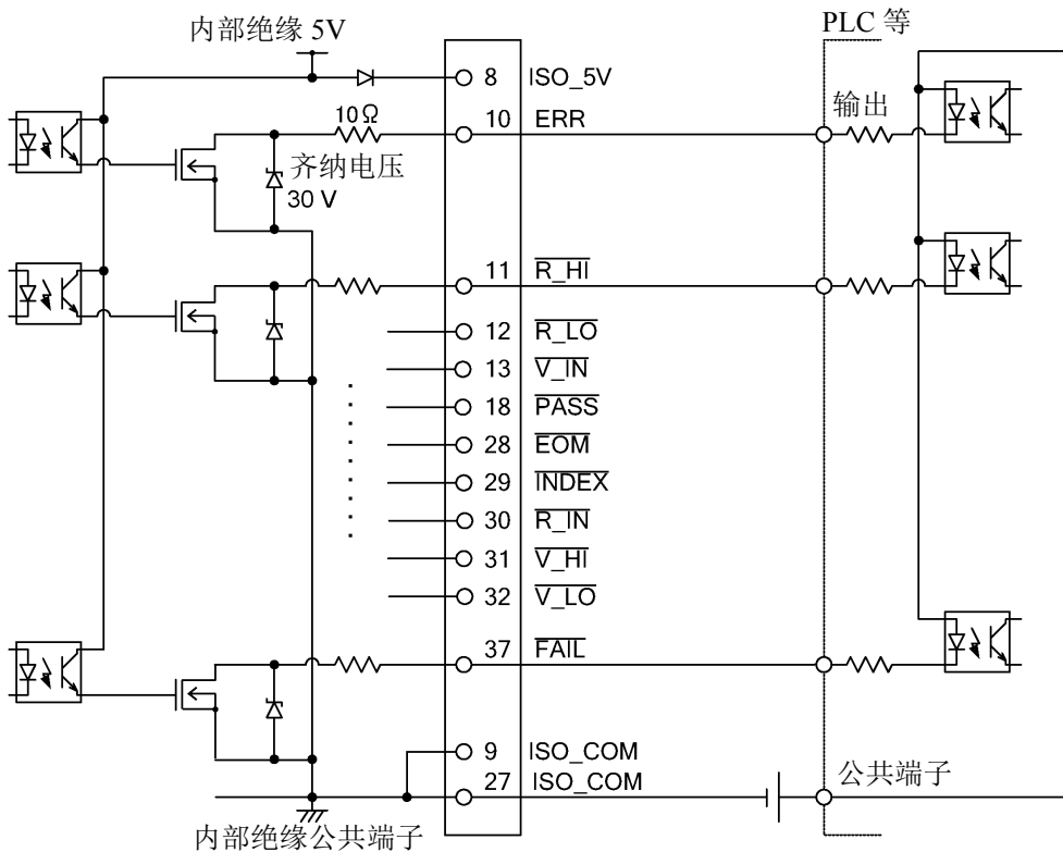
输出电路
