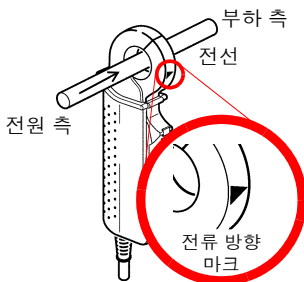
9660 클램프 온 센서
