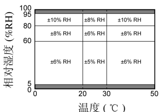
湿度精度表
