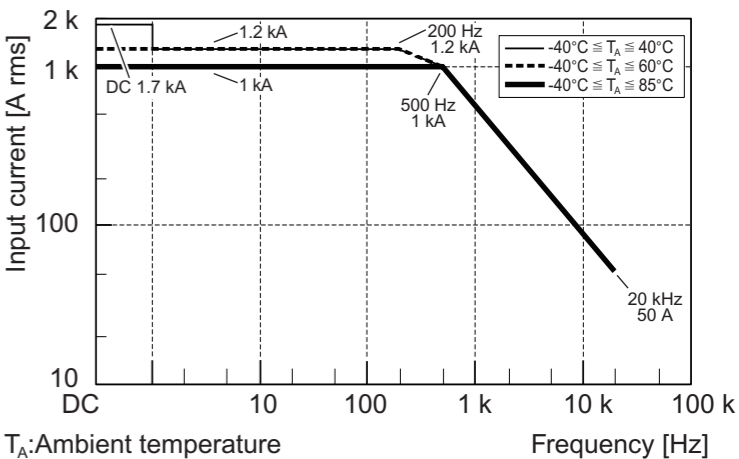
频率降额特性图
