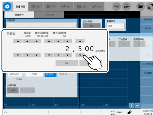
例：任意输入记录长度时
