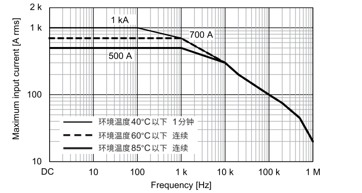
图1. 频率额定值降低特性
