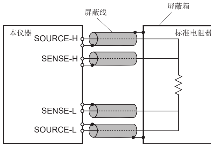
图. 与标准电阻器的连接
