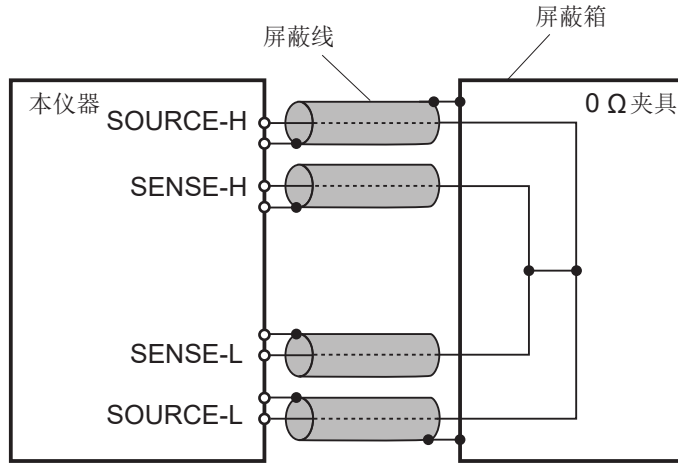
图. 0 Ω 的校正
