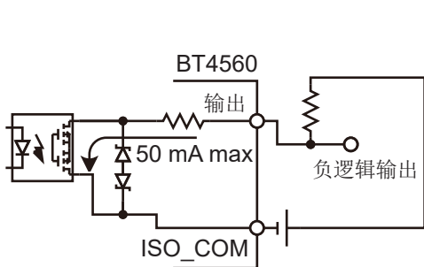
负逻辑输出
