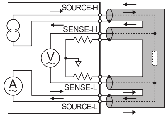
图. 4端子对构造
