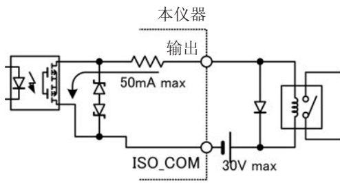
与继电器的连接
