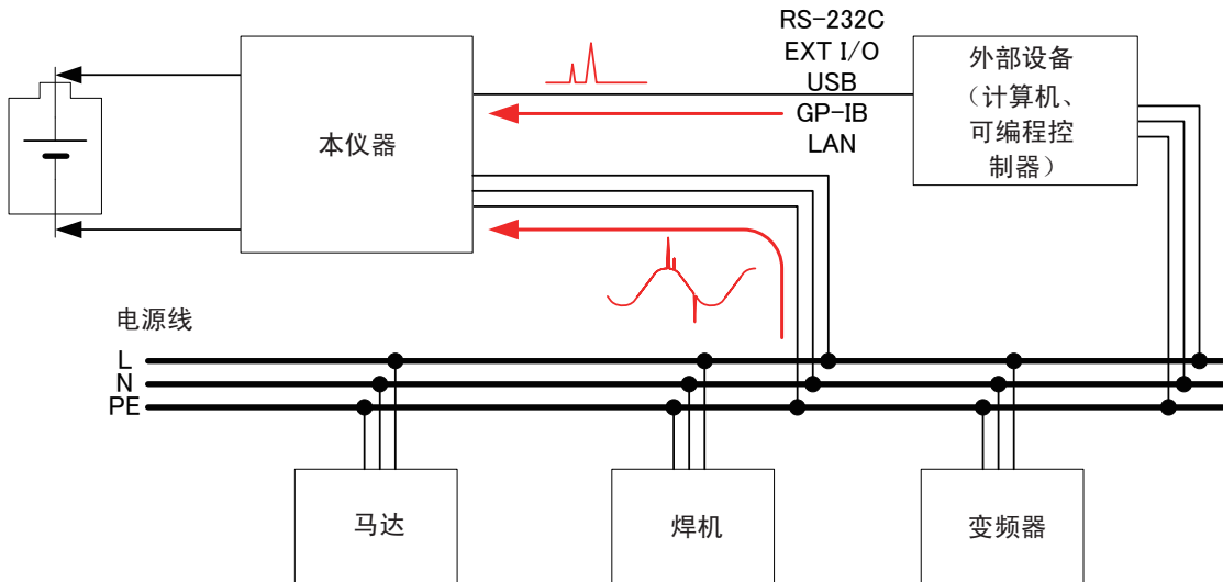
图1. 传导性噪音的进入
