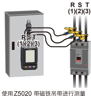
使用 Z5020 带磁铁吊带进行测量
