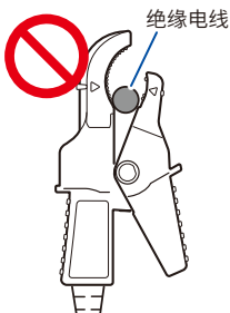
用线夹根部夹住绝缘电线
