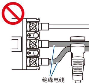
同时夹住电压不同的绝缘电线
