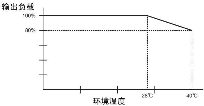
[ 输出特性图 ]
