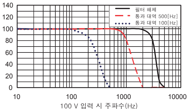
필터 사용 시 주파수 특성의 예 (AC 전압 600.0 V 레인지, 100 V 입력)
