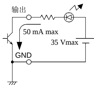
与 LED 的连接
