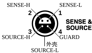
INPUT B 端子 (EPL.0S.304.HLN LEMO 公司制)
