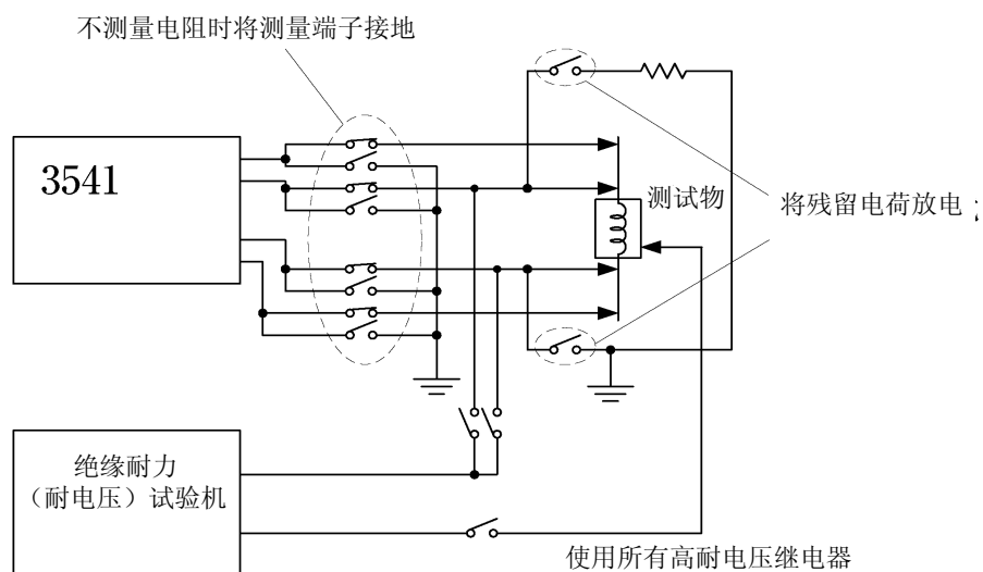
与绝缘耐力试验机的组合
