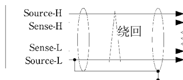
图 3. 低电流电阻测量时
