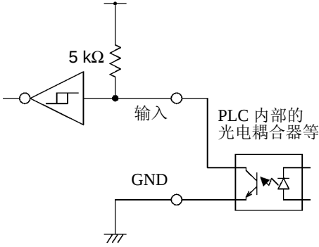
与光电耦合器的连接
